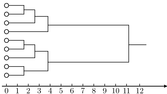
Рис. 8.4: Дендрограма з відстанями.
