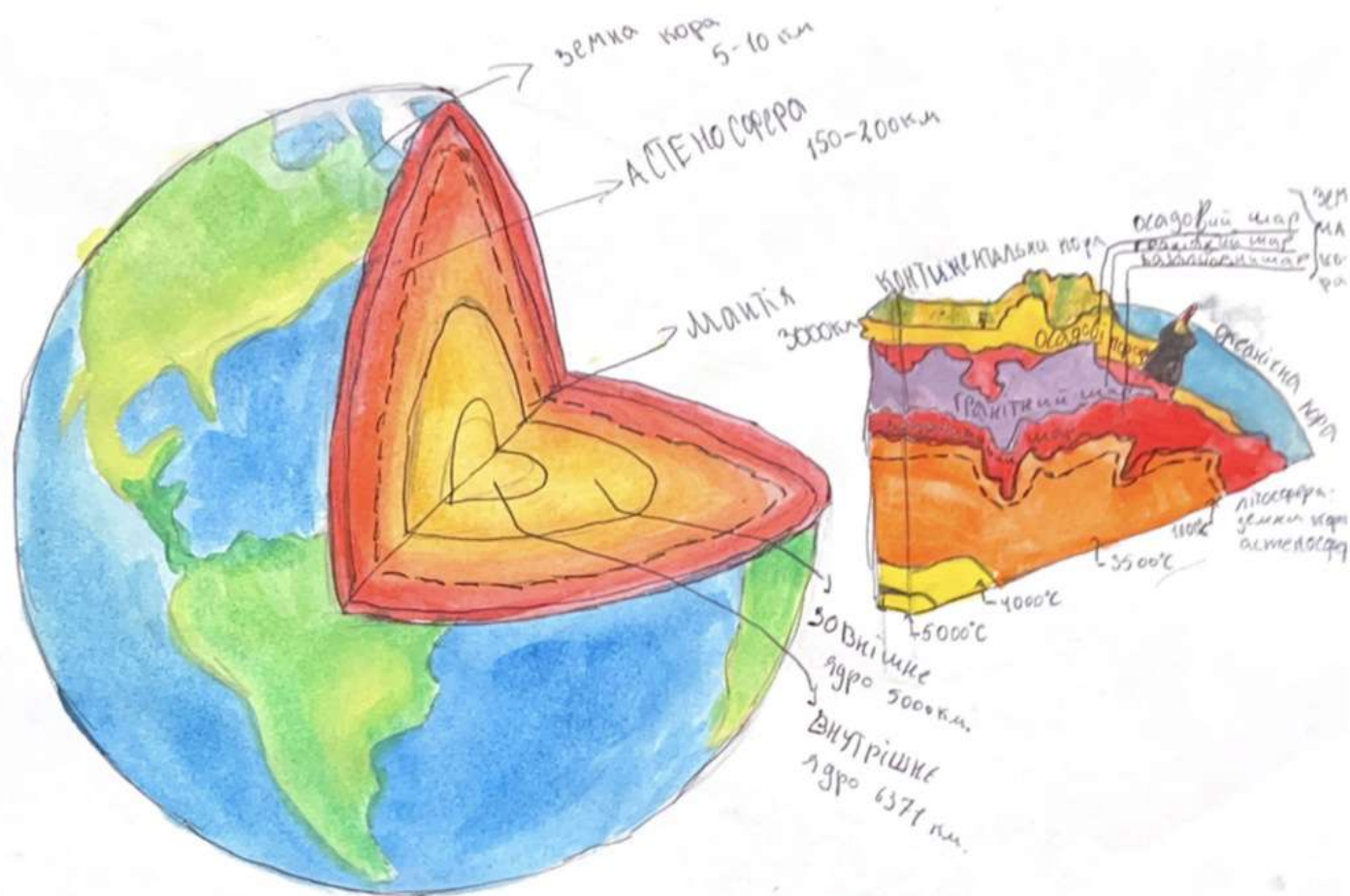
ВНУТРІШНЯ БУДОВА ЗЕМЛІ
