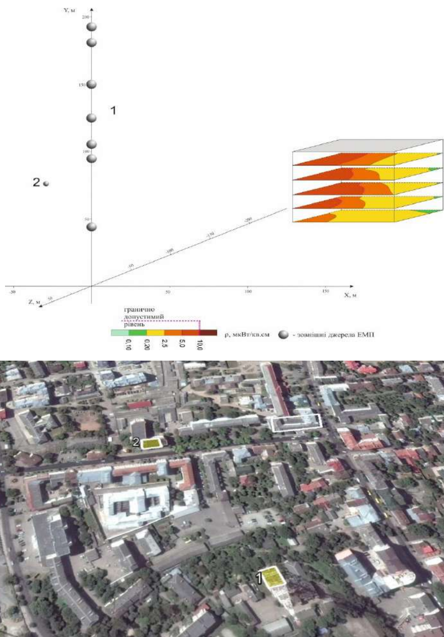
Рисунок 4.9 – Схема поширення ЕМП за показником поверхневої густини потоку енергії, \text{мкВт/см}^2 , на території обласного перинатального центру
