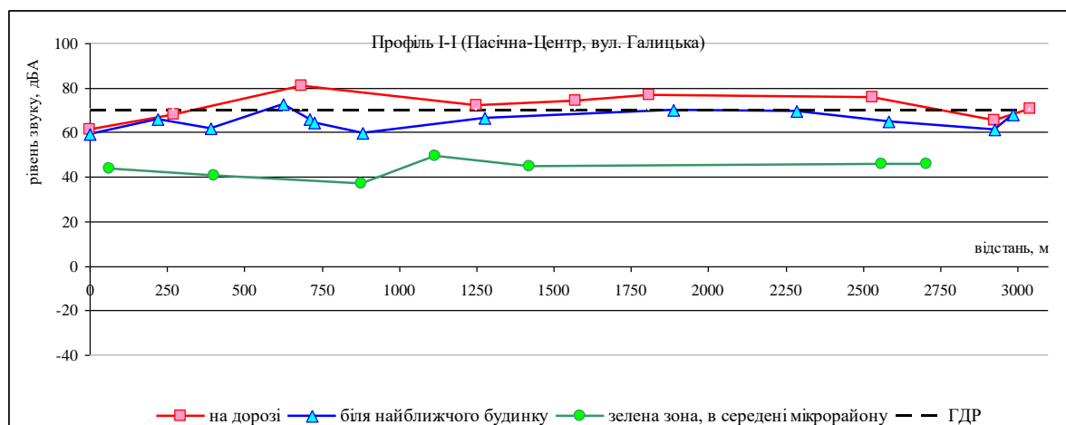
Рисунок 4.2 - Динаміка максимального рівня звуку вздовж профілю 1 «Пасічна-Центр-вул.Галицька»» (поруч зелена зона Парк ім.Воїнів Інтернаціоналістів)
