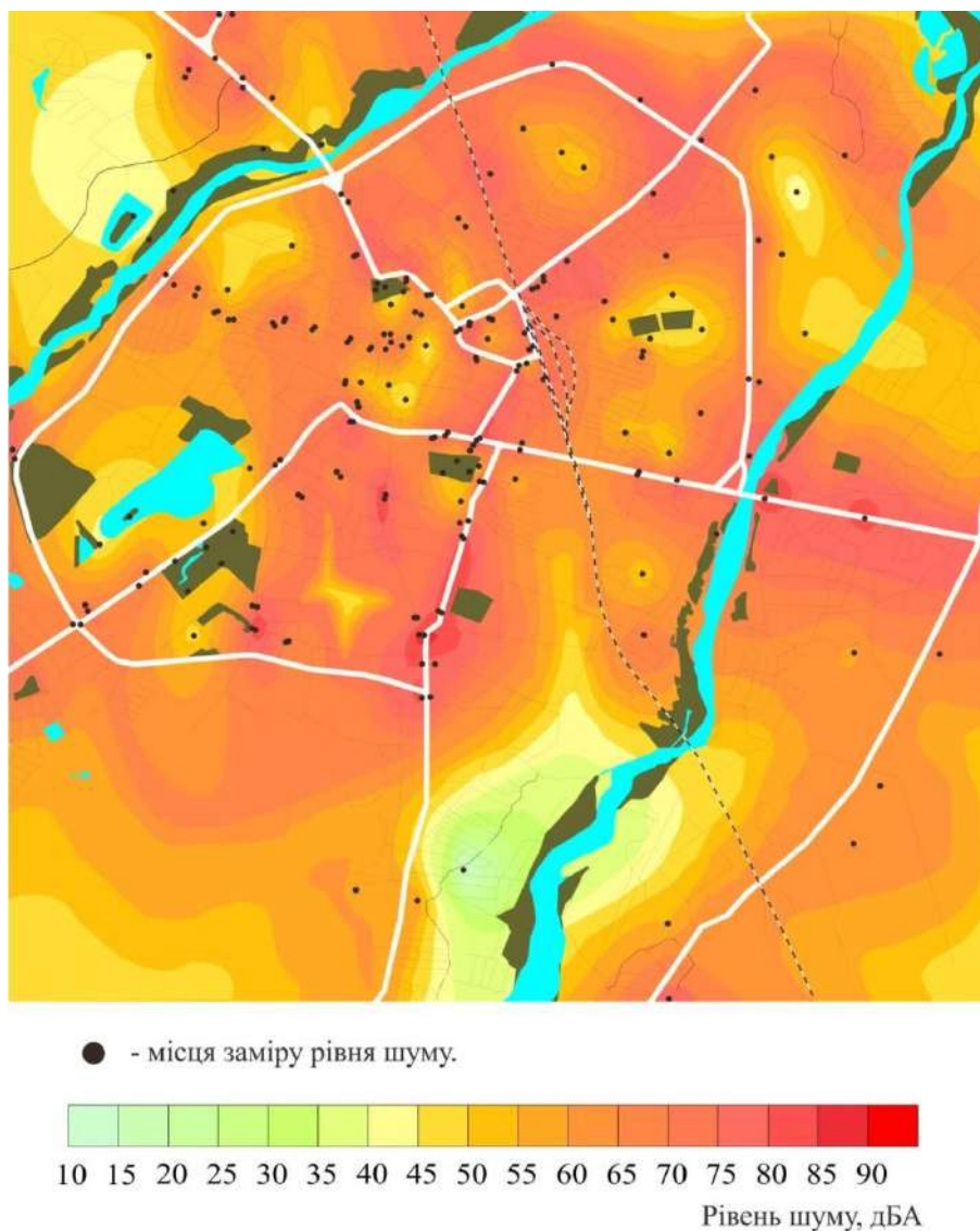
Рисунок 4.4 - Карта акустичного навантаження (карта шуму) на території урбосистеми м.Івано-Франківська [148]
